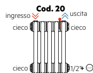
Allacciamenti dall'alto e diaframma saldato
