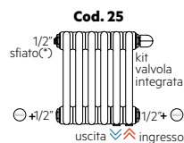
Allacciamento 50 mm con valvola integrata alta
