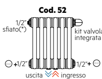
Allacciamento con valvola integrata alta e allacc. idraulici centrali 50 mm (n. minimo di elem. = 6)
