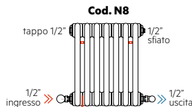
Allacciamenti dal basso con diaframma mobile
