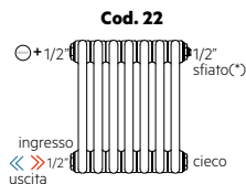
Allacciamento monotubo
