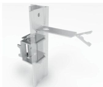
Falso telaio brevettato con sistema di assemblaggio ad incastro
