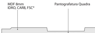
SEZIONE PANTOQUADRA
