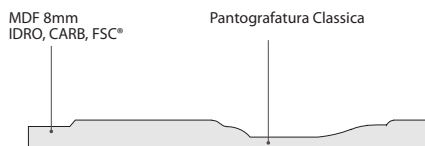
SEZIONE PANTOCLASSICA
