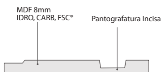
SEZIONE PANTOINCISA
